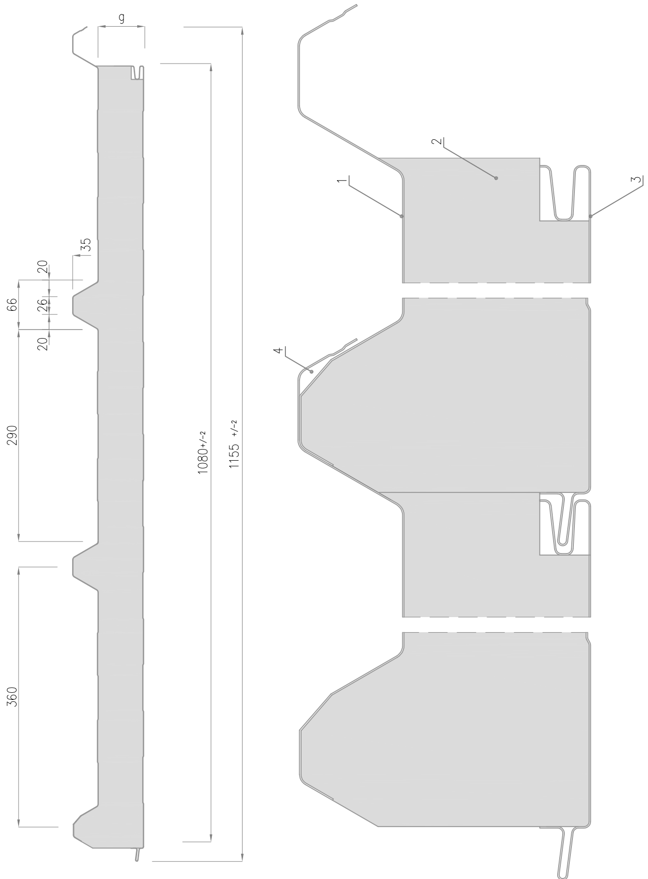
Kuva 4.3. IzoRoof EPS – kattoelementti, ydin EPS
