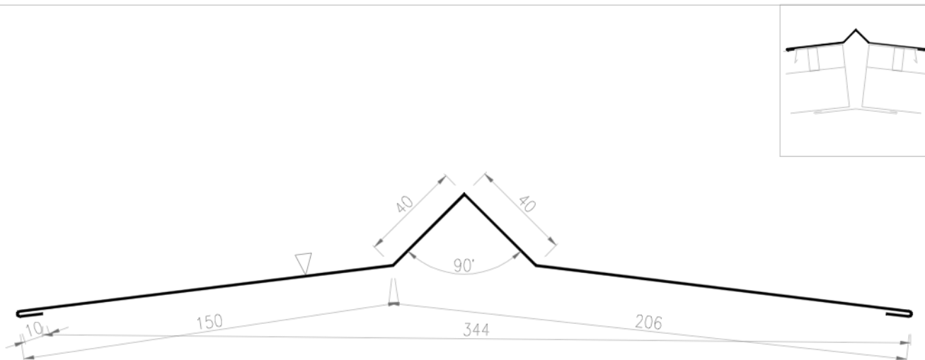
Kuva 41. Harjapelti Ob-03
