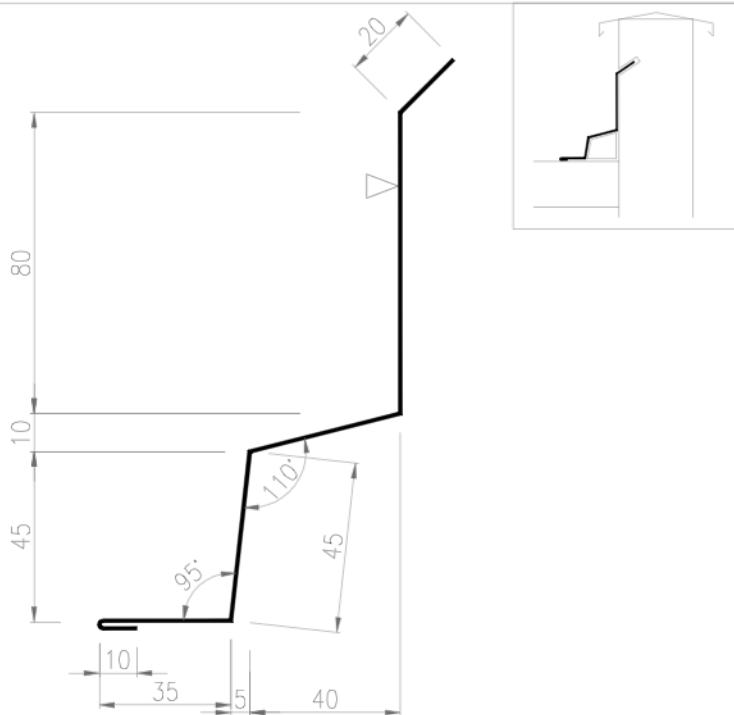
Kuva 57. Korkean päätyseinän leikatun elementin tippalista, Ob-22
