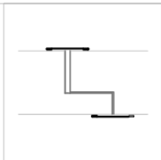
Kuva 58. Peitelista Ob-23 IzoCold elementtien jatkosauma
